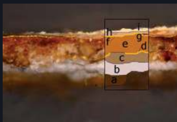
Sezione stratigrafica D
