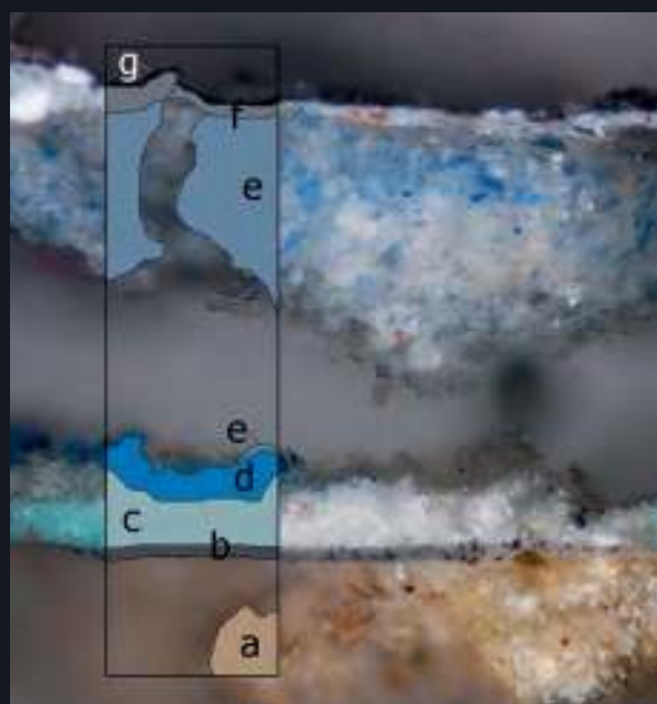
Sezione stratigrafica C
